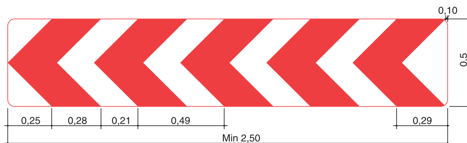
Figur 7. O 41 ”Retningspil” (alle ubenævnte mål er i m)
