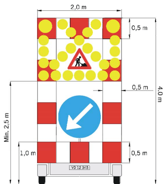
Figur 4. Eksempler på mobil afspærring i standardstørrelser
